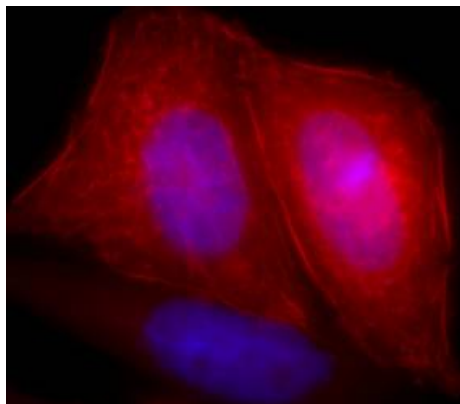
DY-547-Phalloidin
